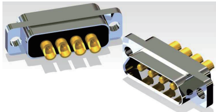
J30J 04P04 0 P 000 S0 000 0
