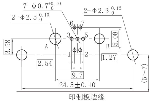
J30J09P02KPW01W10000弯插印制板开孔尺寸
