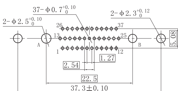
J30J39P02KPN01N10000直插印制板开孔尺寸
