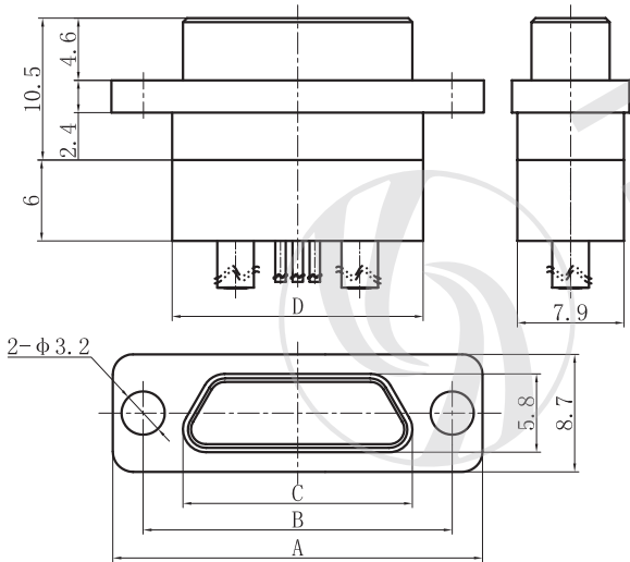
J30J 09P02 J S C00 C0 000 0
