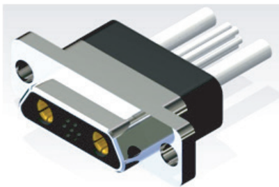
J30J 09P02 J S C00 C0 000 0
