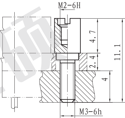
外形尺寸
