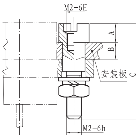
外形尺寸
