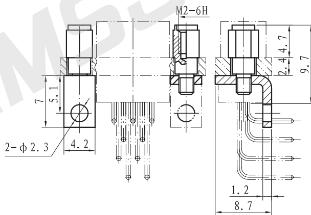
外形尺寸
