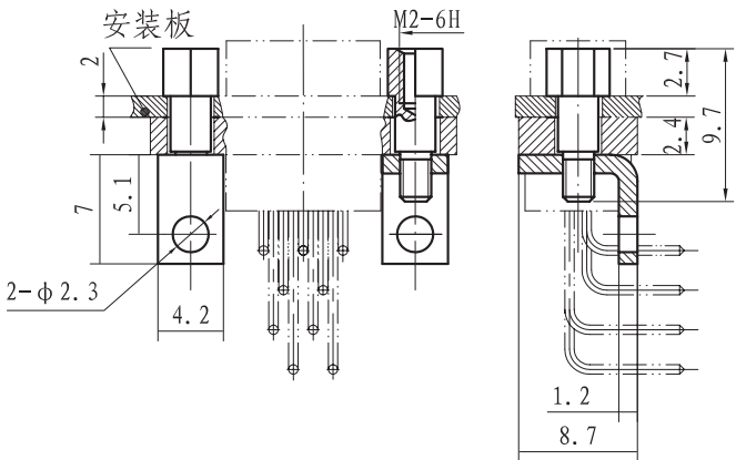
外形尺寸
