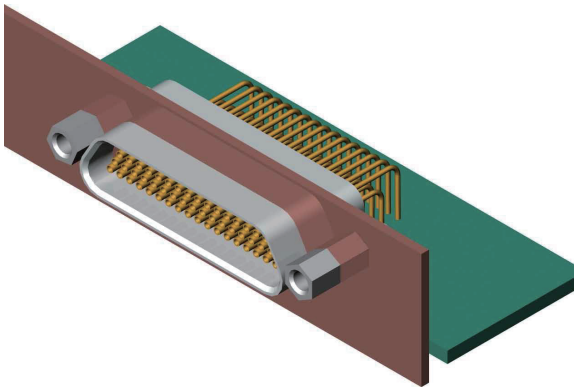
组装示意图
