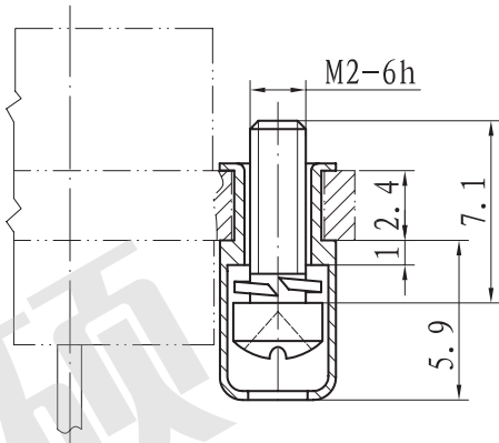
外形尺寸
