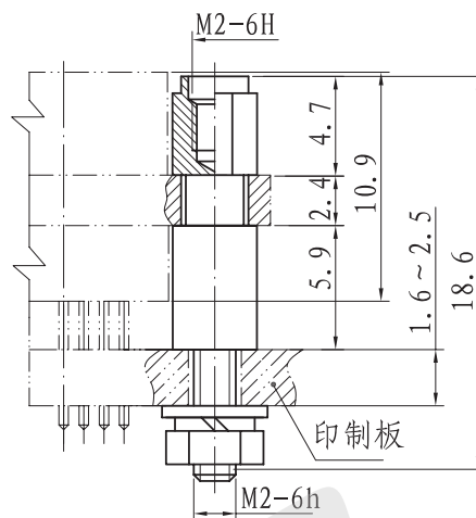
外形尺寸
