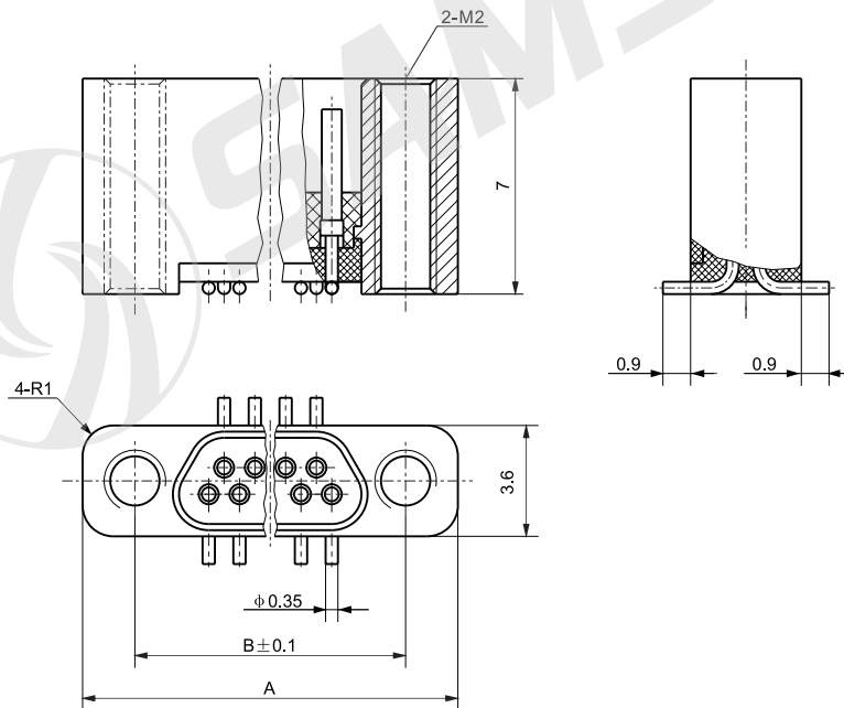
产品外形尺寸图
