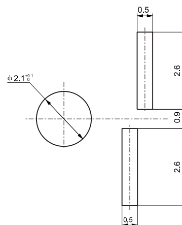
引脚封装尺寸局部放大图
