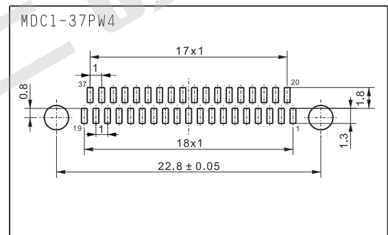
引脚封装尺寸局部放大图
