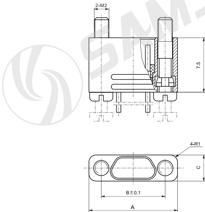
产品外形尺寸图
