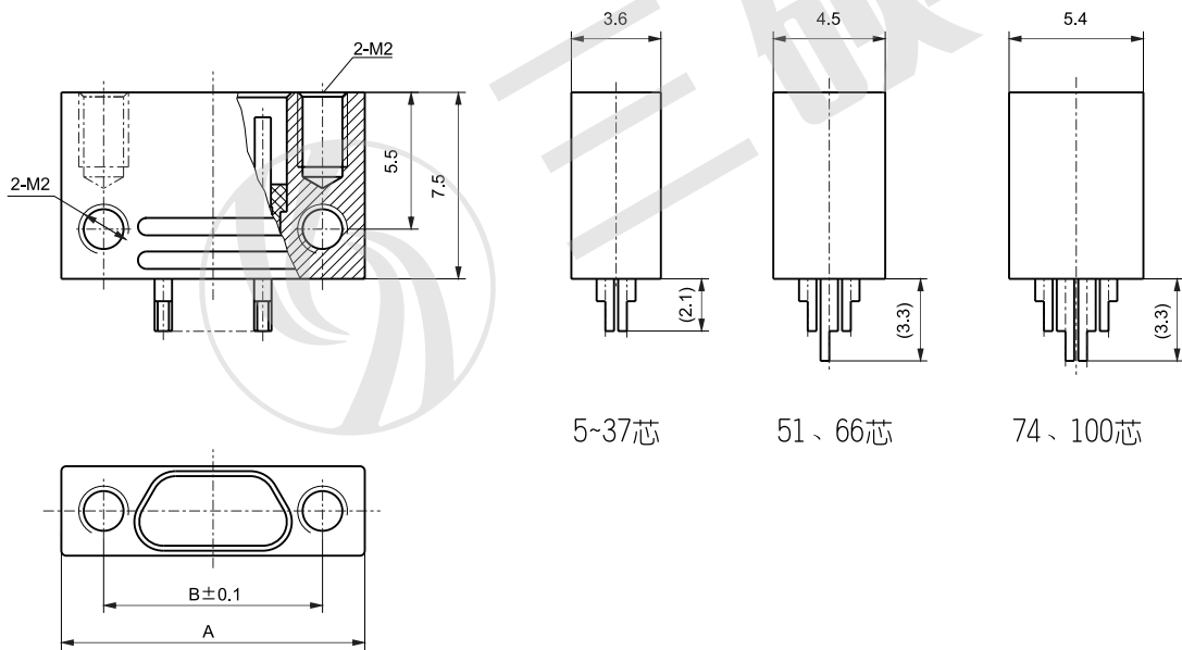
产品外形尺寸图
