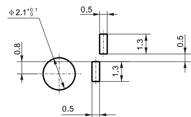
引脚封装尺寸局部放大图
