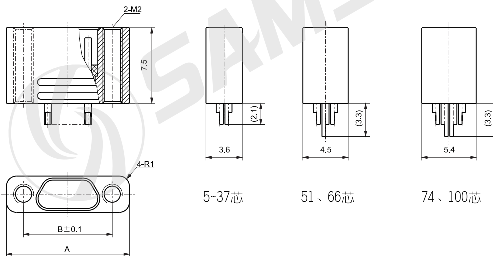
产品外形尺寸图
