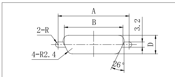
板后安装开孔尺寸 (100 芯除外)
