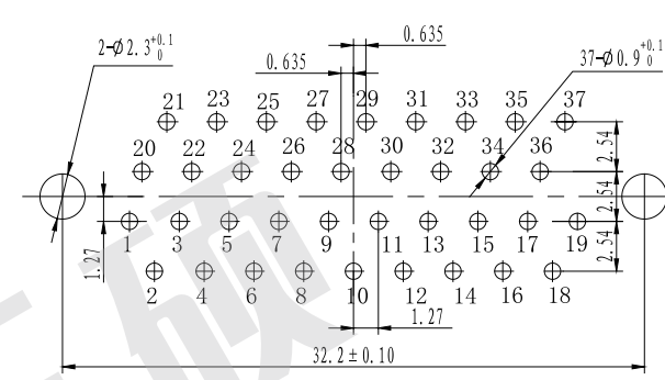
J30J-37ZKN、ZKN3、ZKN4
