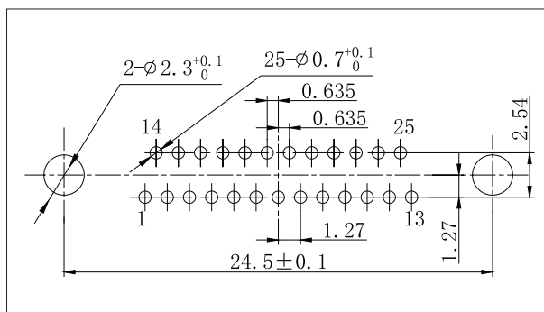
J30J-25ZKN-J、ZKN4-J
