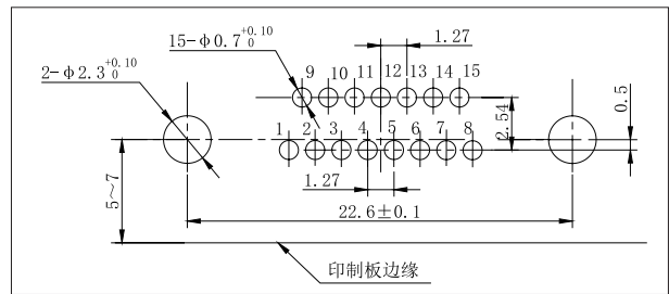
J30JA-15ZKW-J
