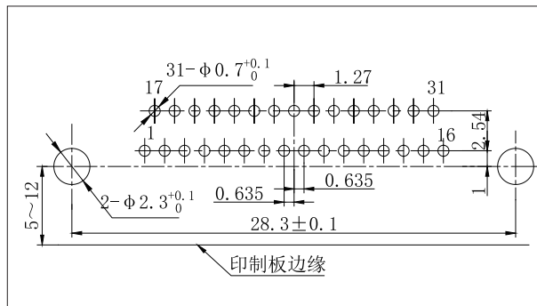
J30J-31ZKW-J
