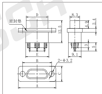
J30JM-74 ~ 100ZKS
