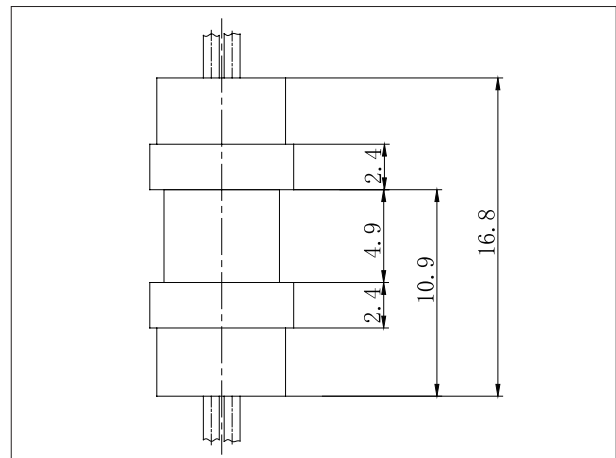
左视图
