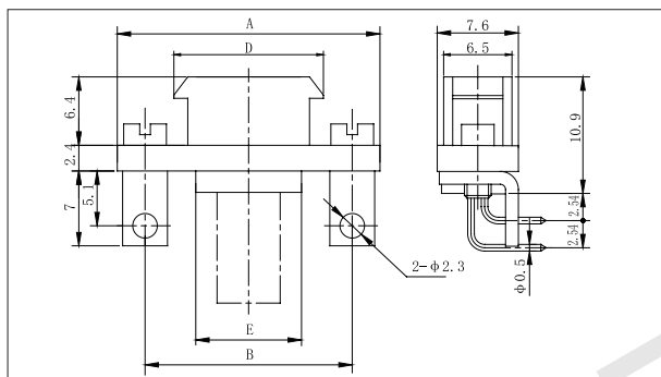
J30JA-9 ~ 37ZKW-J
