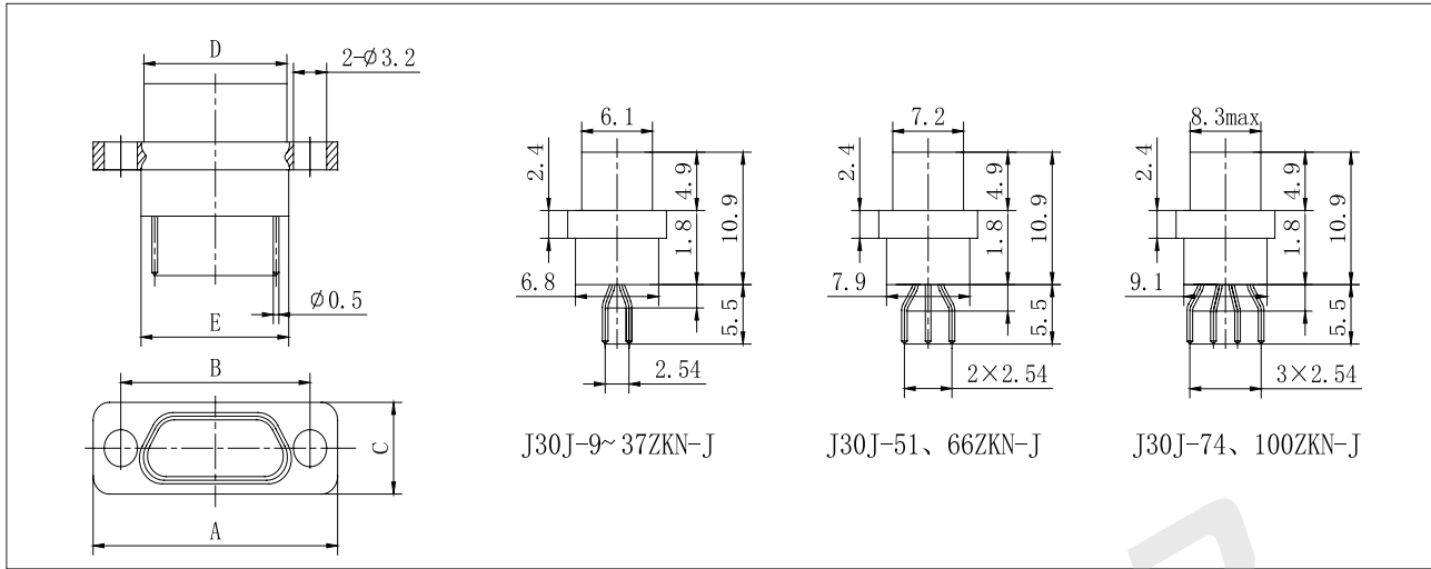
产品外形尺寸图
