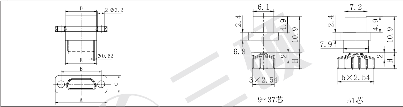
J30J-9~51ZKN3/J30J-9~51ZKN4
