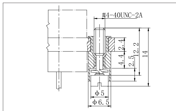
产品外形尺寸图
