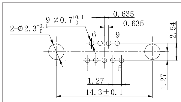
J30J-9ZKN-J、ZKN4-J
