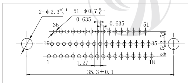
J30JA-51ZKN-J
