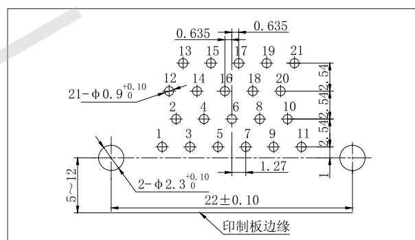
J30J-21ZKW
