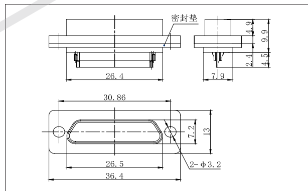
J30JM1-51ZKS
