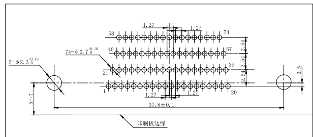
J30JA-74ZKW-J
