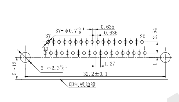
J30J-37TJW-J
