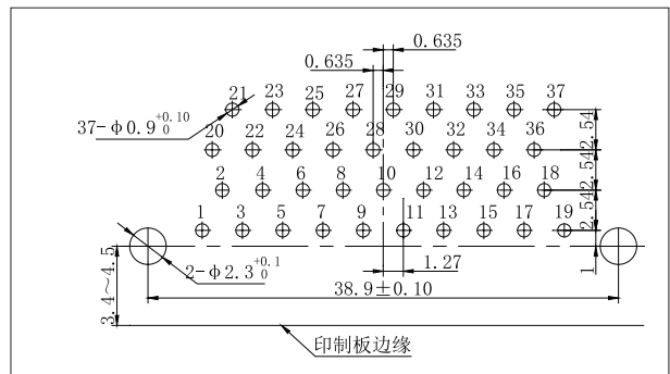
J30JC-37ZKW-Q
