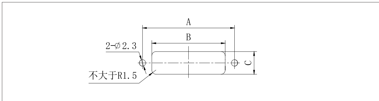
板前安装开孔尺寸
