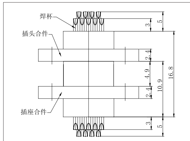
J30J-51~100 芯
