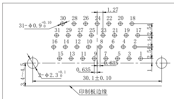
J30J-31TJW-Q8
