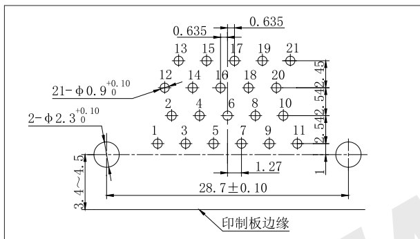
J30JC-21ZKW-Q
