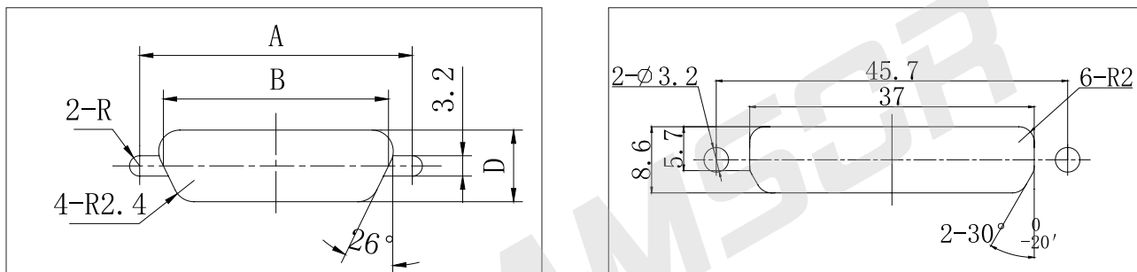
板后安装开孔尺寸 (100 芯除外)
