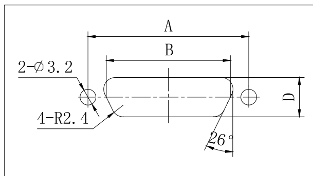
板后安装开孔尺寸 (100 芯除外)
