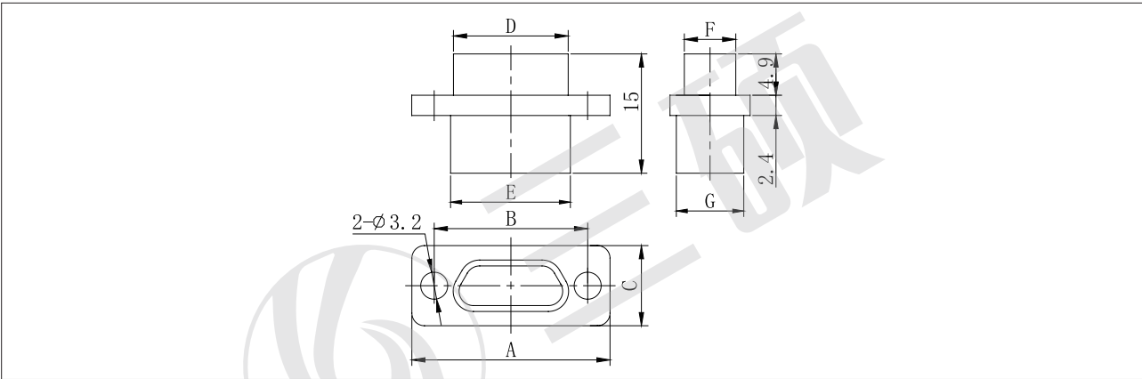
产品外形尺寸图
