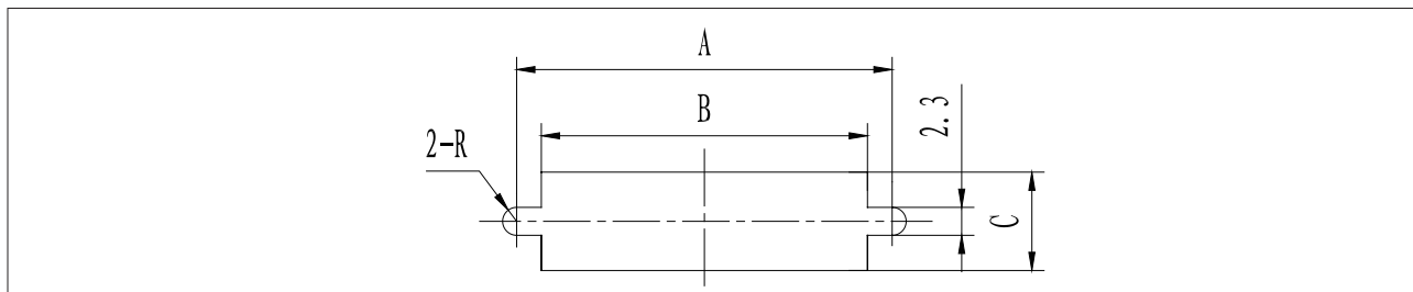
板前安装开孔尺寸
