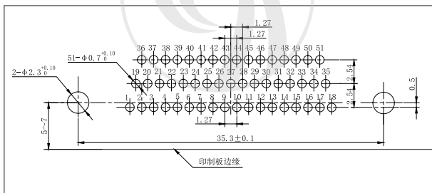
J30JA-51ZKW-J
