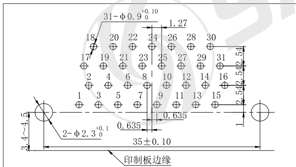
J30JC-31ZKW-Q
