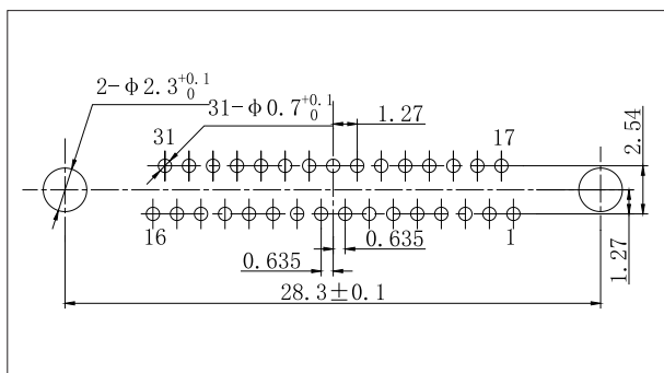
J30J-31TJN-J
