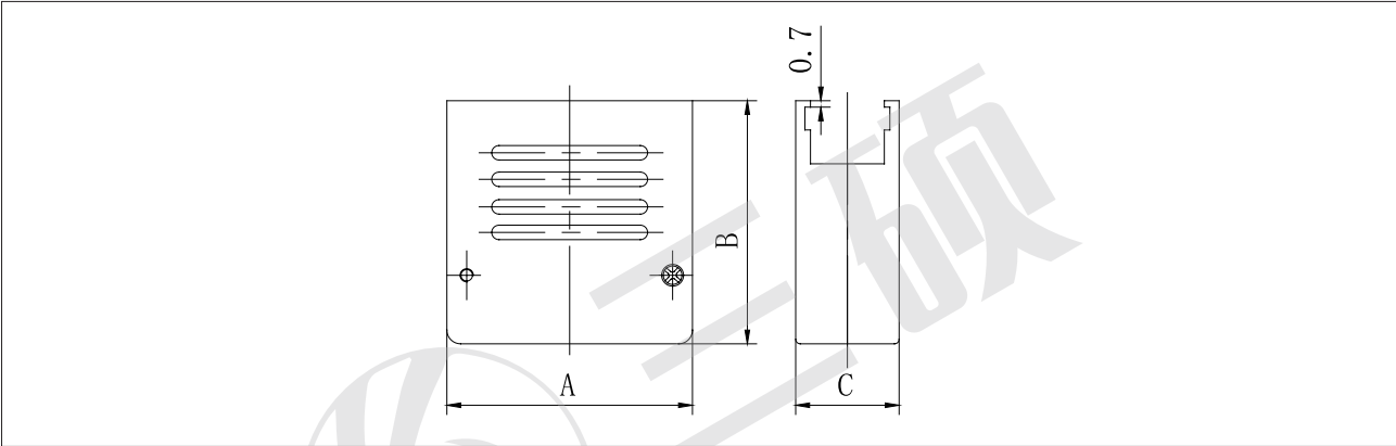
J30J- □ A2 线夹合件
