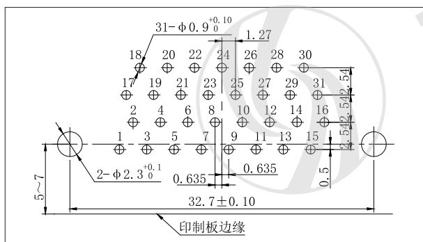
J30JA-31ZKW
