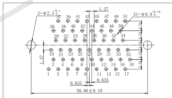
J30J-51ZKN、ZKN3、ZKN4
