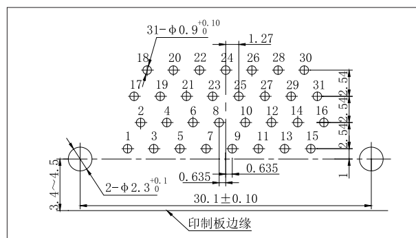
J30J-31ZKW-Q8
