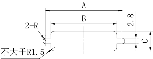
板前安装开孔尺寸
