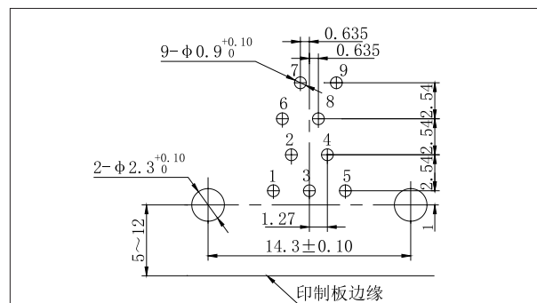
J30J-9ZKW
