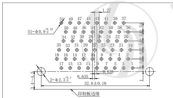
J30J-51TJW-Q8
