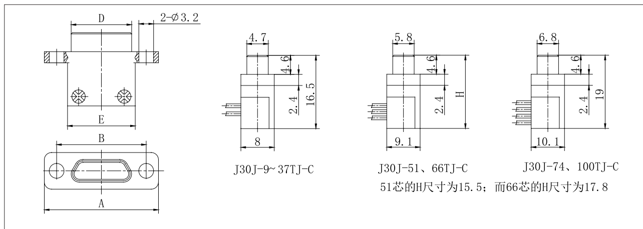
各芯数插头合件左视图
