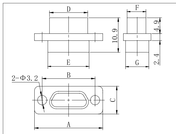
J30J- □ ZK
