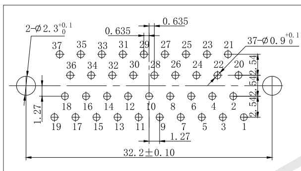
J30J-37TJN、TJN4、TJN8
