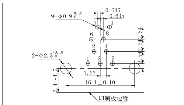
J30J-9ZKW-Q8
