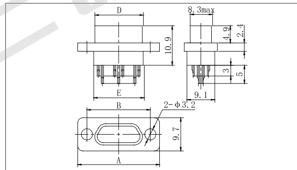
J30J-74, 100ZKS
