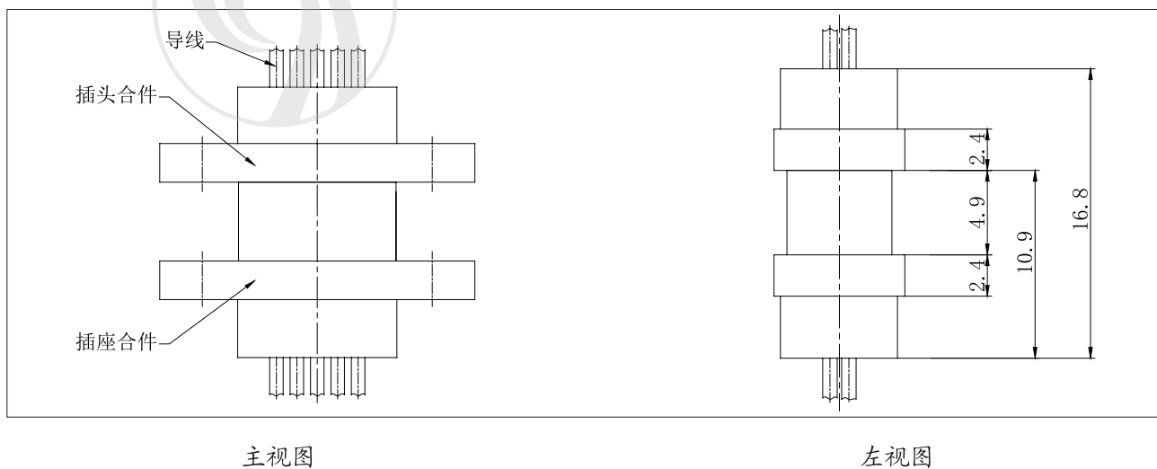
产品对接图
