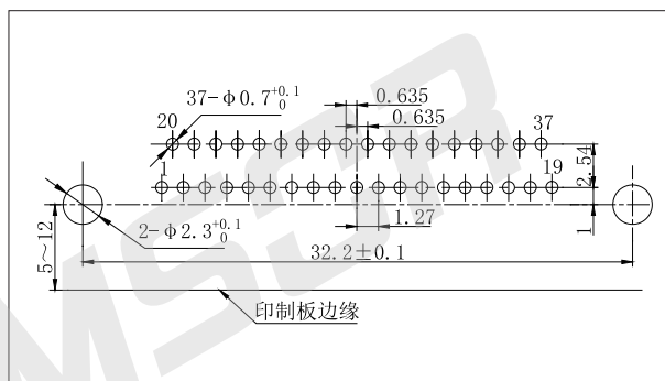
J30J-37ZKW-J
