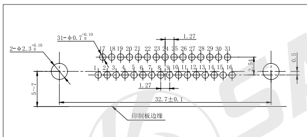
J30JA-31ZKW-J
