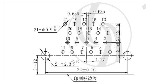
J30J-21TJW
