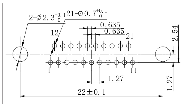
J30J-21ZKN-J、ZKN4-J
