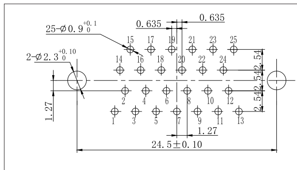
J30J-25ZKN、ZKN3、ZKN4
