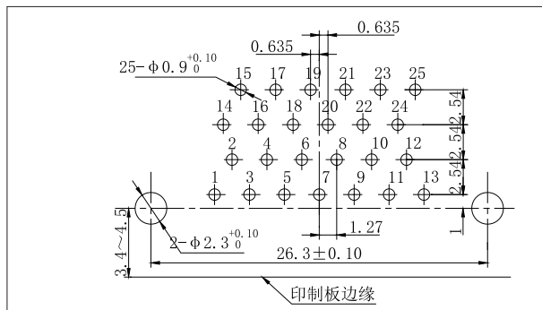
J30J-25ZKW-Q8
