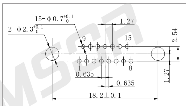
J30J-15ZKN-J、ZKN4-J
