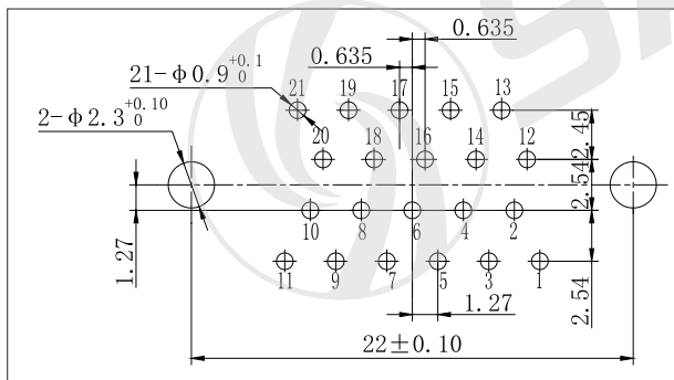
J30J-21TJN、TJN4、TJN8
