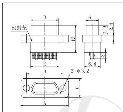
J30JM-9 ~ 37ZKS
