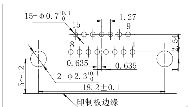
J30J-15TJW-J
