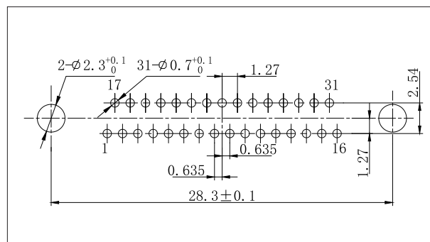
J30J-31ZKN-J、ZKN4-J
