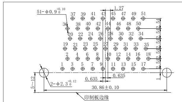
J30J-51ZKW
