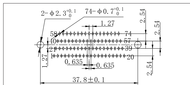
J30JA-74ZKN-J
