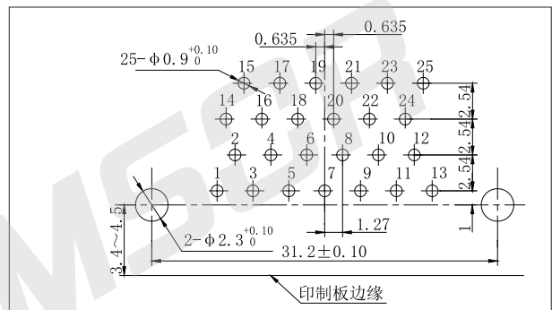
J30JC-25ZKW-Q
