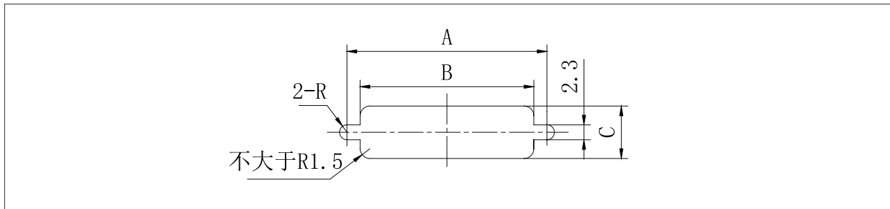
板前安装开孔尺寸
