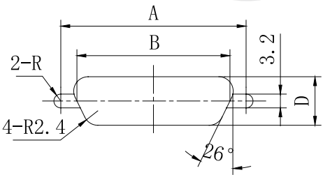
板后安装开孔尺寸 (100 芯除外)
