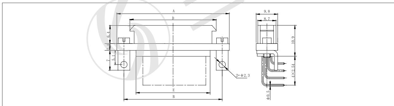
J30JA-74、100ZKW-J
