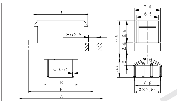
J30JA-9 ~ 37ZKN
