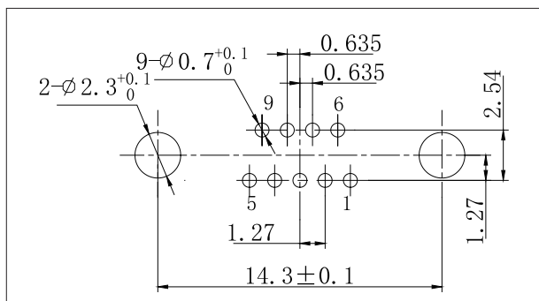
J30J-9TJN-J
