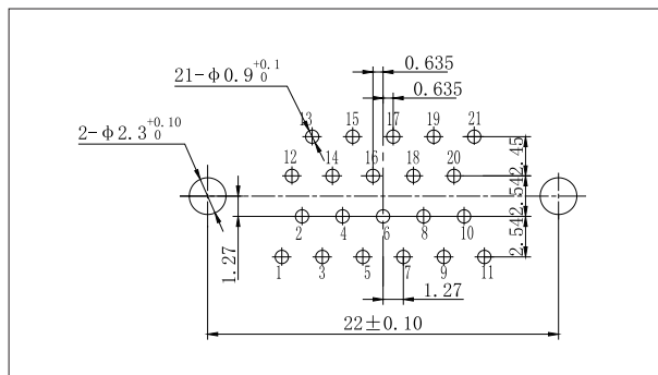
J30J-21ZKN、ZKN3、ZKN4
