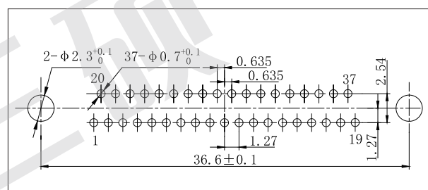
J30JA-37ZKN-J
