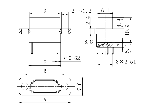
J30J-9~37ZKN
