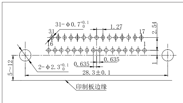
J30J-31TJW-J
