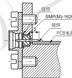
安装示意图
