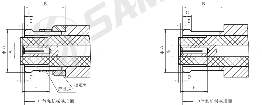
※ 可插入直径为 \phi 0.38 \pm 0.03 的插针。 SMP 系列插孔接触件连接器界面
