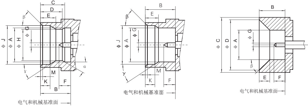
SMP 系列插针接触件连接器界面 (全擒纵或有限擒纵)
