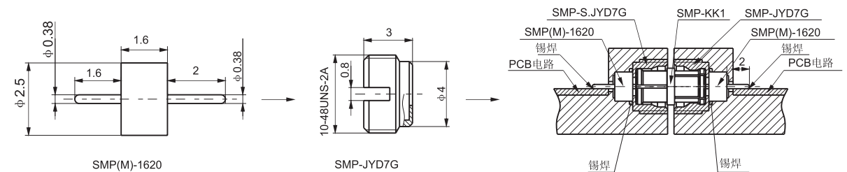
安装示意图
