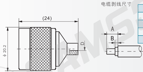
电缆剥线尺寸
