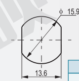
建议安装开孔尺寸
