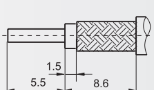
电缆剥线尺寸
