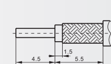
电缆剥线尺寸
