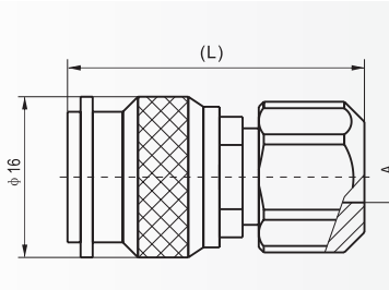
电缆剥线尺寸
