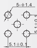
建议安装开孔尺寸
