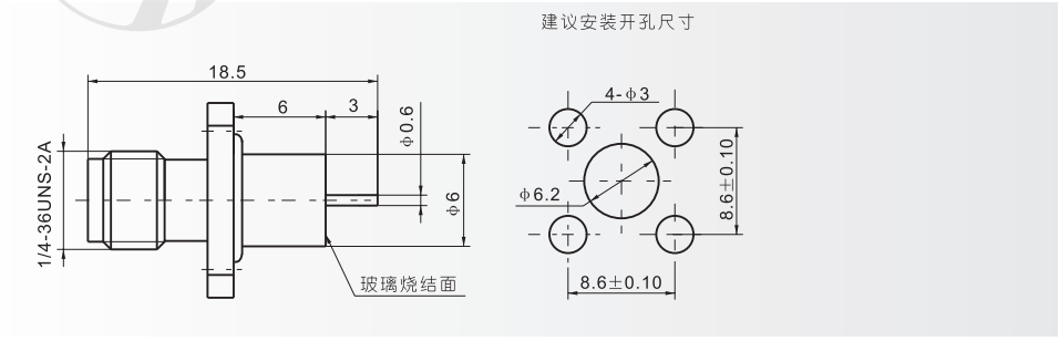
SMA(M)-KFD16(气密封)
