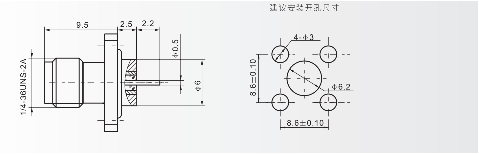
SMA(M)-KFD17(气密封)
