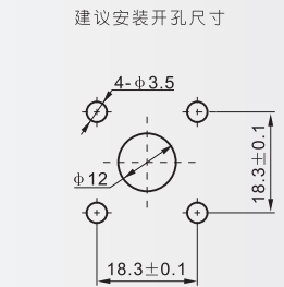
建议安装开孔尺寸
