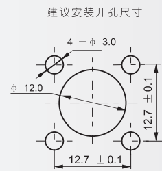
建议安装开孔尺寸
