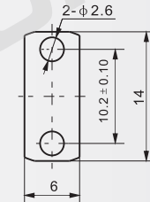
法兰盘尺寸
