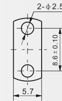
法兰盘尺寸
