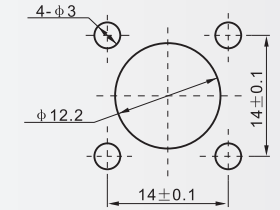
建议安装开孔尺寸
