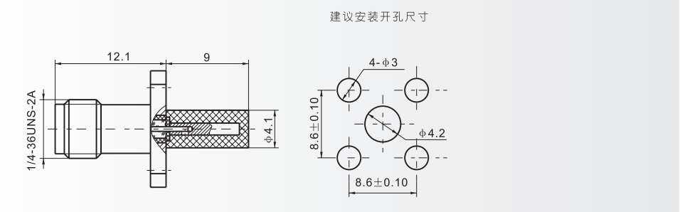
SMA(M)-KFD15(气密封)
