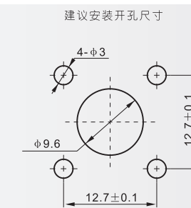
建议安装开孔尺寸
