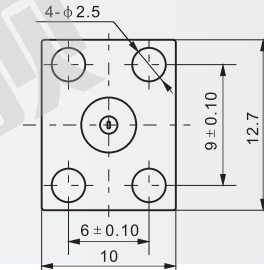
法兰盘尺寸
