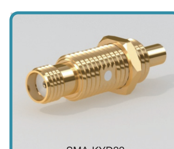
SMA-KYD22
