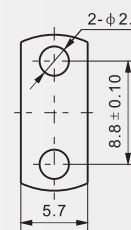
法兰盘尺寸
