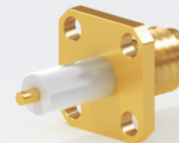
SMA-KFD225
