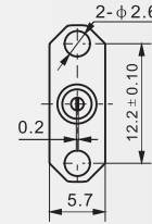
法兰盘尺寸
