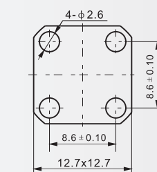
法兰盘尺寸
