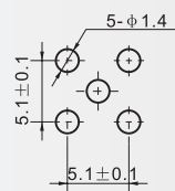
建议安装开孔尺寸
