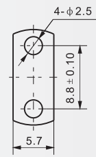
法兰盘尺寸
