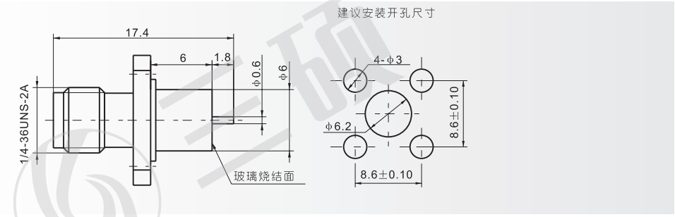
SMA(M)-KFD14(气密封)
