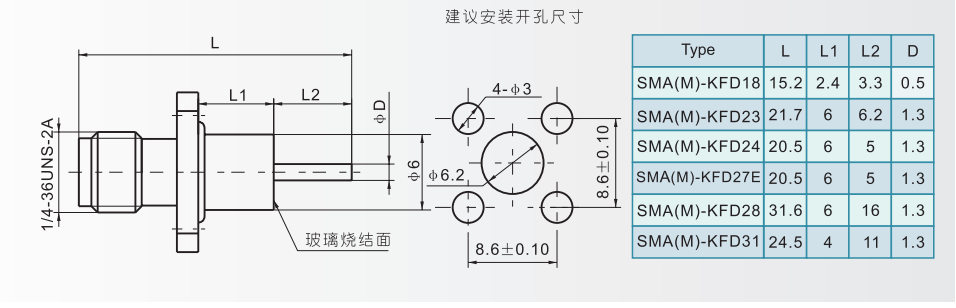
SMA(M)-KFD18等(气密封)
