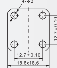
法兰盘尺寸
