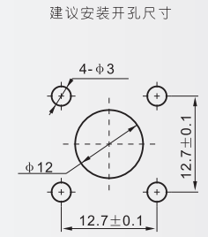
建议安装开孔尺寸
