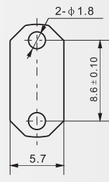
法兰盘尺寸
