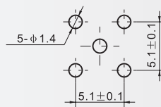
建议安装开孔尺寸
