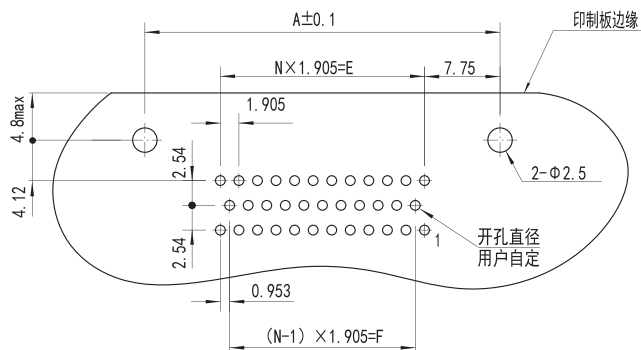
弯式带安装耳印制板插座（A向）
