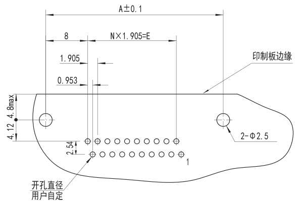
弯式带安装耳印制板插座 (A向)
