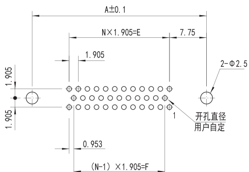
直式带安装耳印制板插座（A向）
