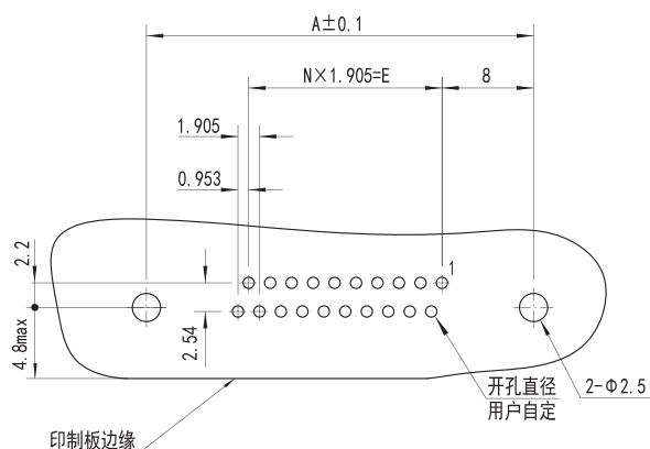
弯式带安装耳印制板插头 (A向)
