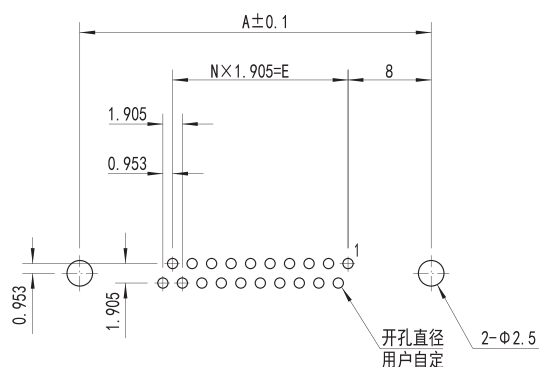
直式带安装耳印制板插头 (A向)
