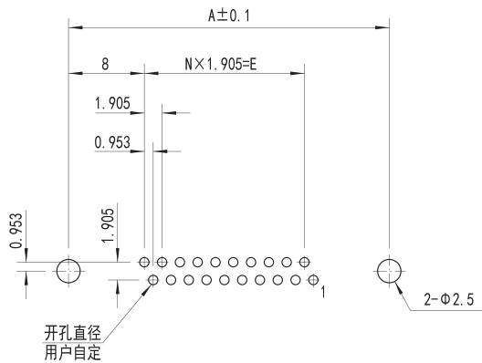
直式带安装耳印制板插座 (A向)
