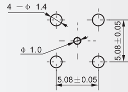
建议安装开孔尺寸
