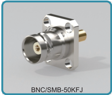
BNC/SMB-50KFJ
