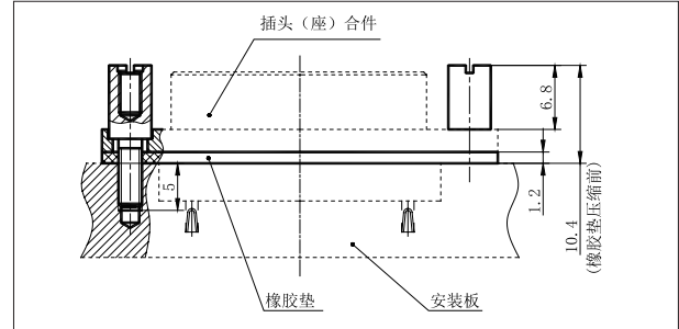
外形尺寸图
