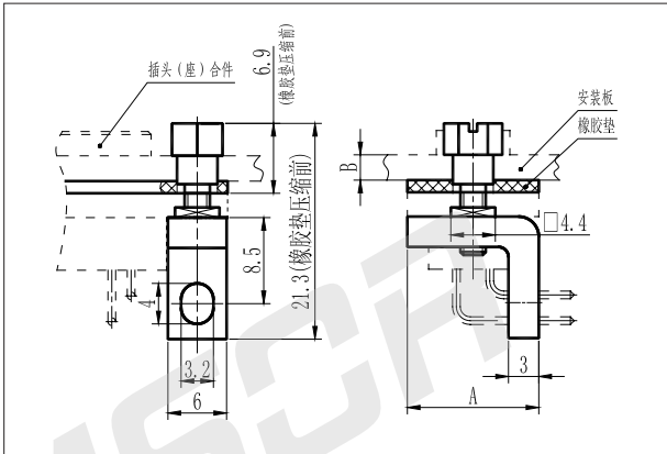
外形尺寸图
