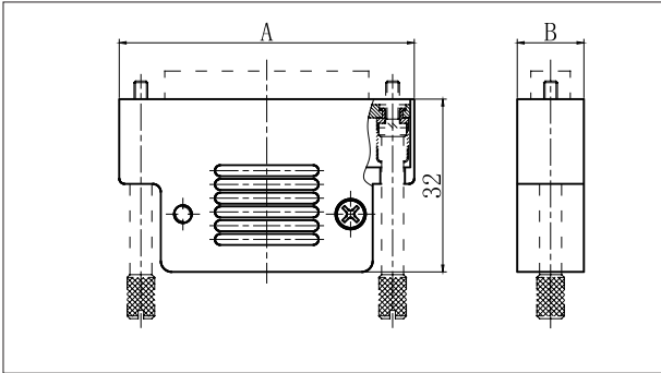
D 型尾罩合件外形尺寸图
