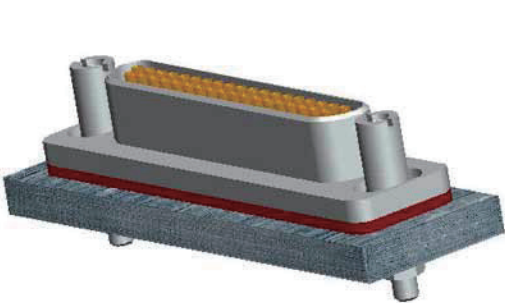
安装示意图
