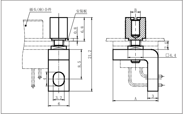
外形尺寸图
