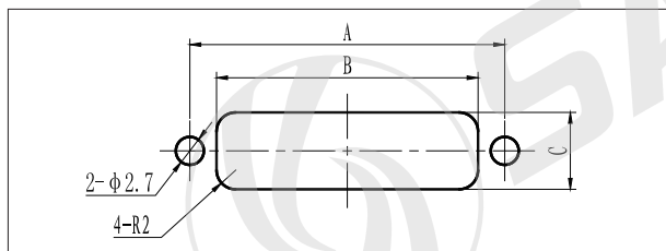
板前安装板开孔尺寸
