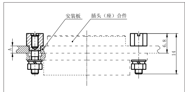
外形尺寸图
