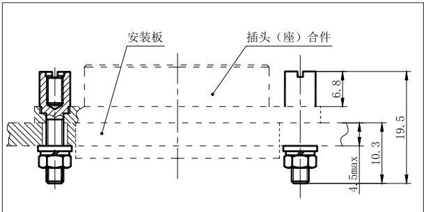
外形尺寸图
