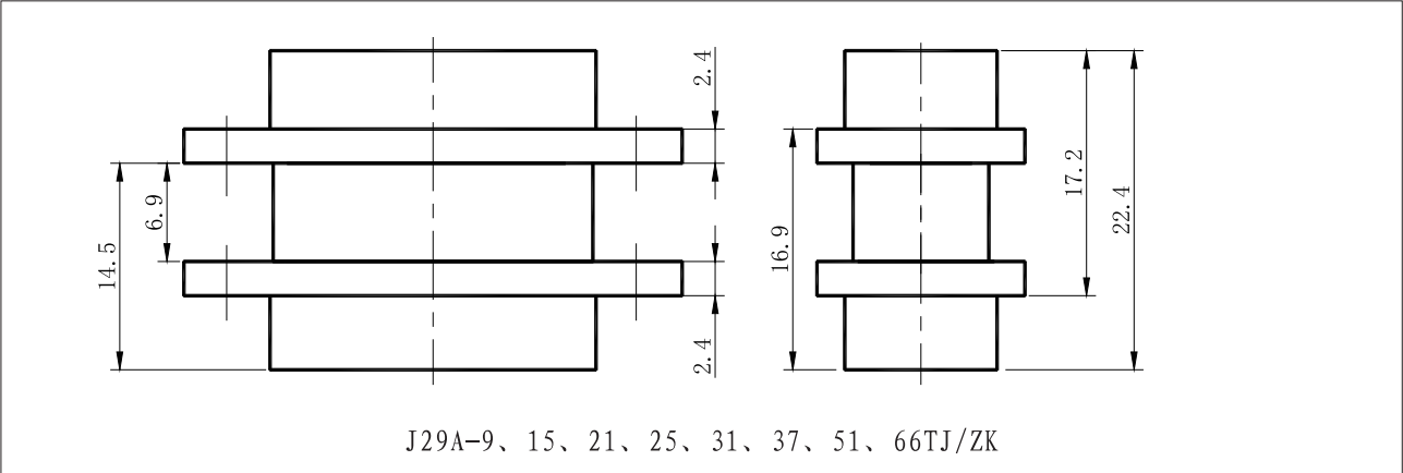
产品对接后外形图
