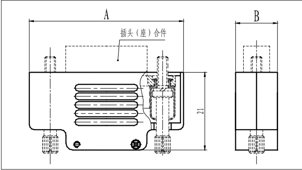
D1 型尾罩合件外形尺寸图
