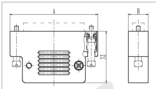
D2 型尾罩合件外形尺寸图
