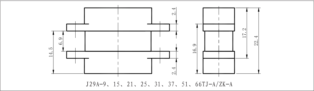
产品对接后外形图
