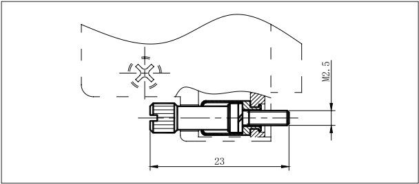
外形尺寸图
