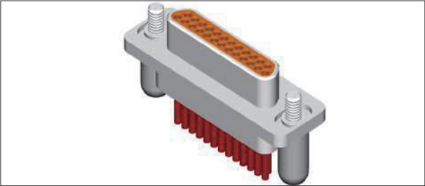
组装示意图
