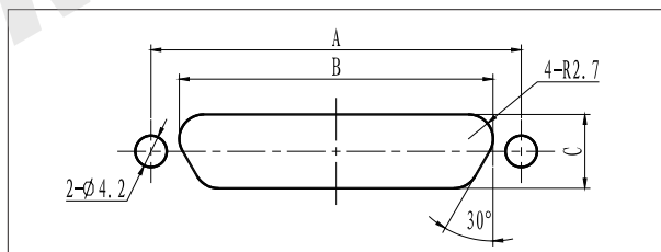
板后安装板开孔尺寸
