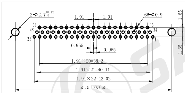
J29A 弯插印制板系列
