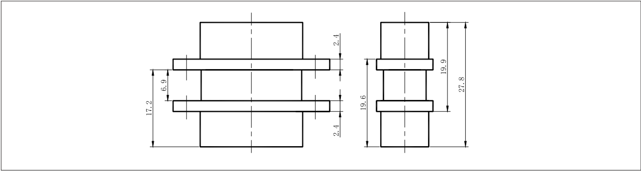
产品对接后外形图
