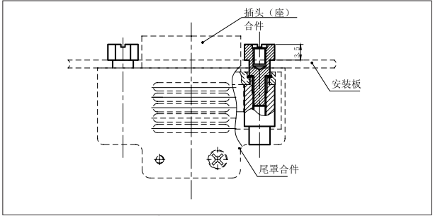
外形尺寸图
